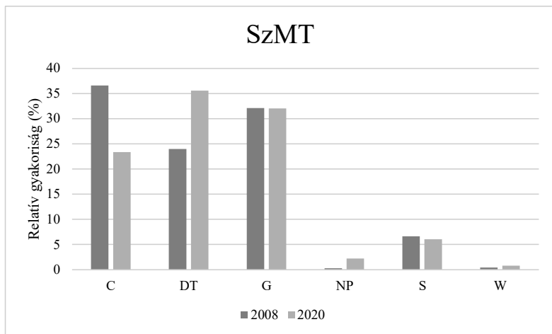
1. ábra: Szociális magatartási típusok relatív gyakoriságának eloszlása
