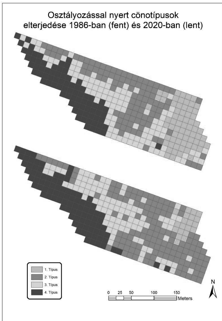
3. ábra: Hierarchikus osztályozással nyert cönotípusok elterjedése 1986-ban (fent) és 2020-ban (lent)
