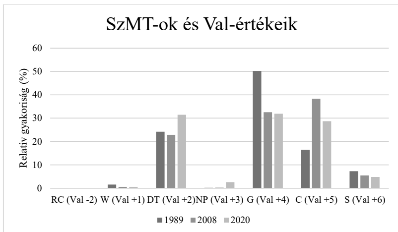
5. ábra: Szociális Magatartási Típusok (SzMT) és Természetességi Értékszámok (Val) relatív gyakoriságának eloszlása a három vizsgált év szerint bontva
