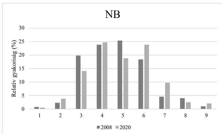
2. ábra: Nitrogén-igény relatív gyakoriságának eloszlása
