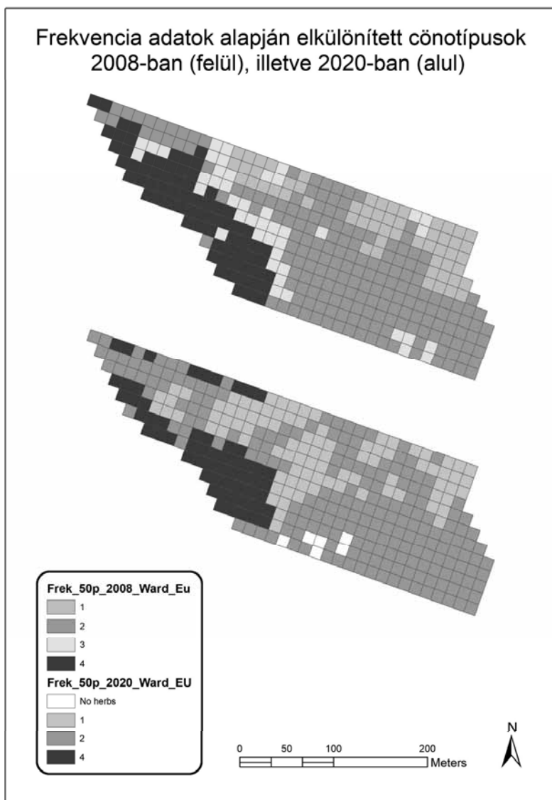
4. ábra: Frekvencia adatok alapján elkülönített cönotípusok 2008-ban (felül) és 2020-ban (alul)
