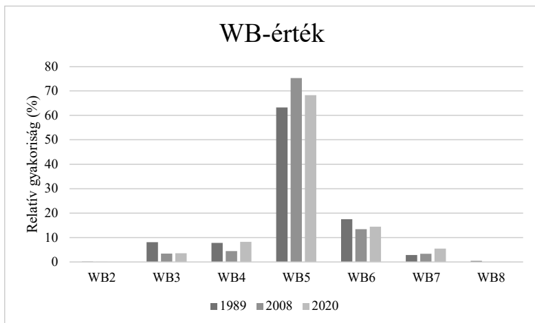
7. ábra: A nedvességigény értékek (WB-érték) relatív gyakoriságának eloszlása a három vizsgált év szerint bontva
