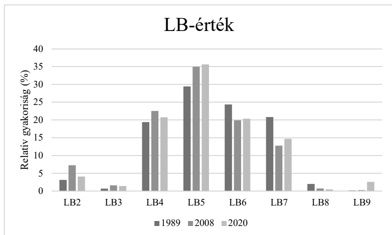
6. ábra: A relatív fényigény értékek (LB-érték) relatív gyakoriságának eloszlása a három vizsgált év szerint bontva
